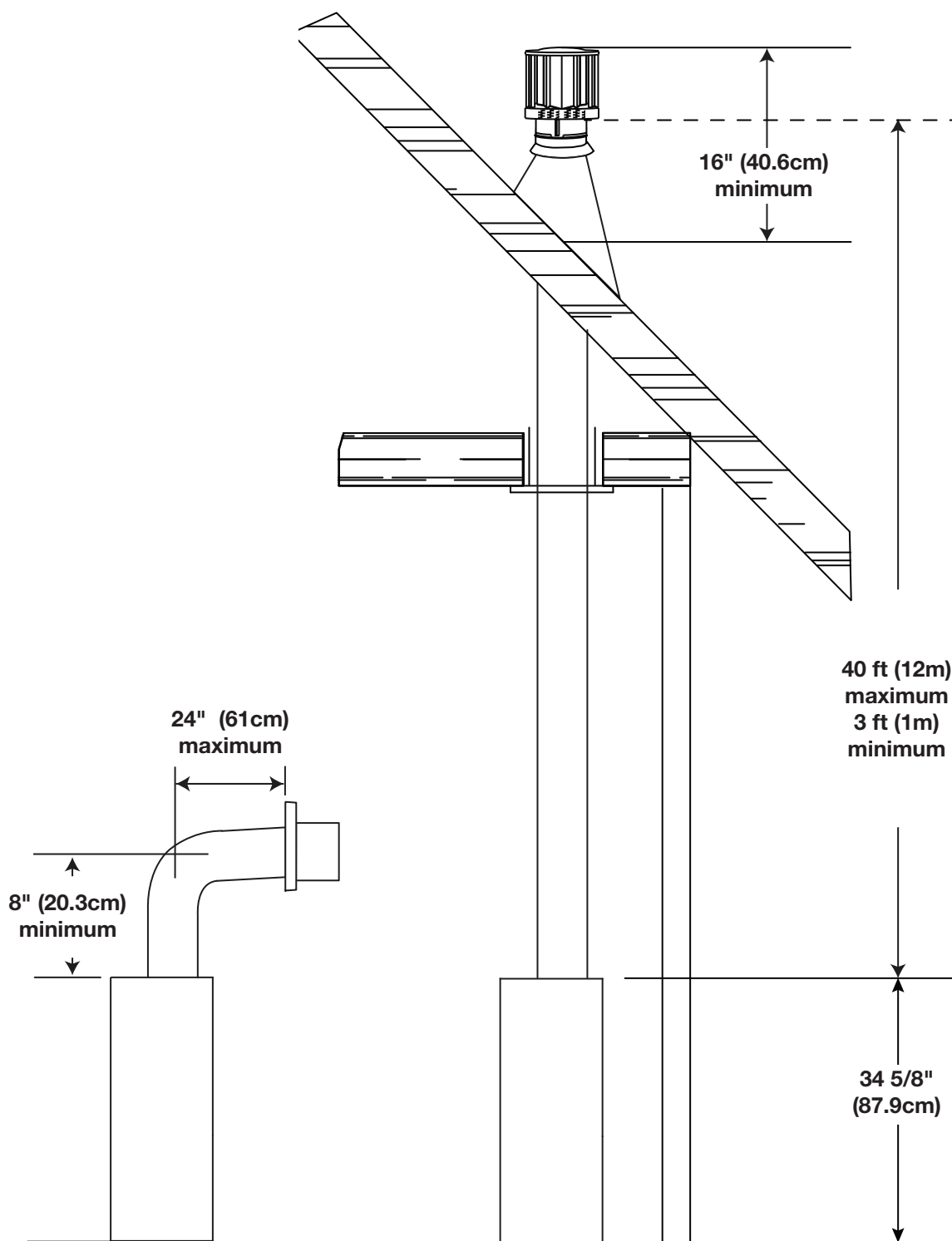
TOP VENT
